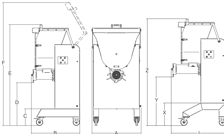
MASTER 90 Y12 optional high legs X: 333 mm / Y: 717 mm Z: 1575 mm / J: 806 mm
